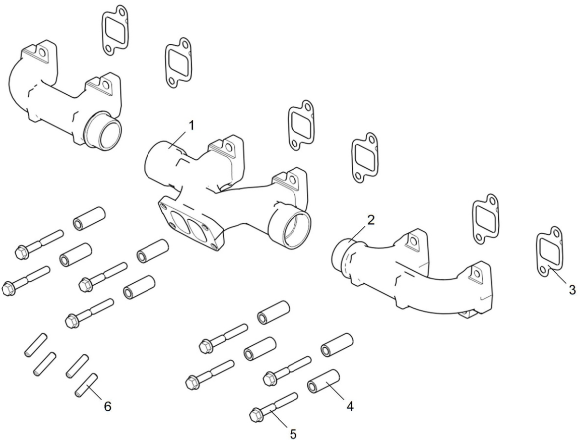
Рисунок 1 Коллектор выпускной
