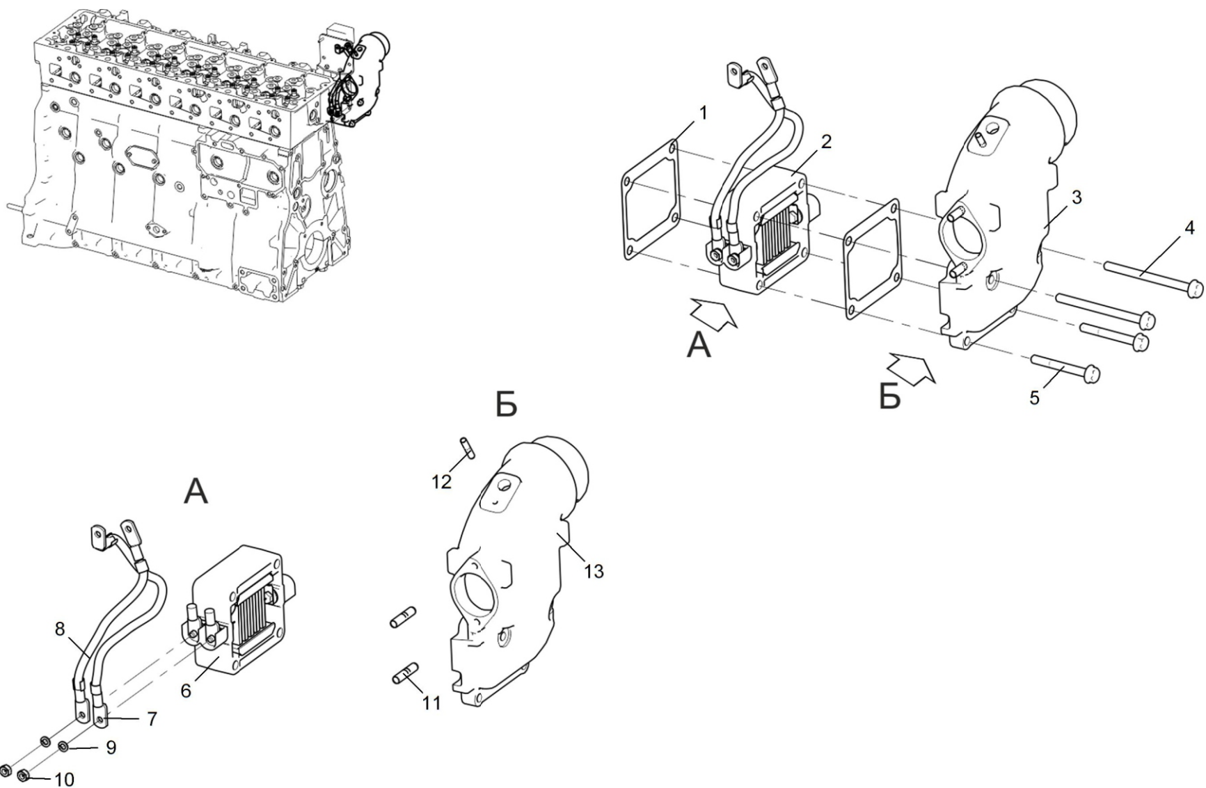
Рисунок 1 Тракт впускной
