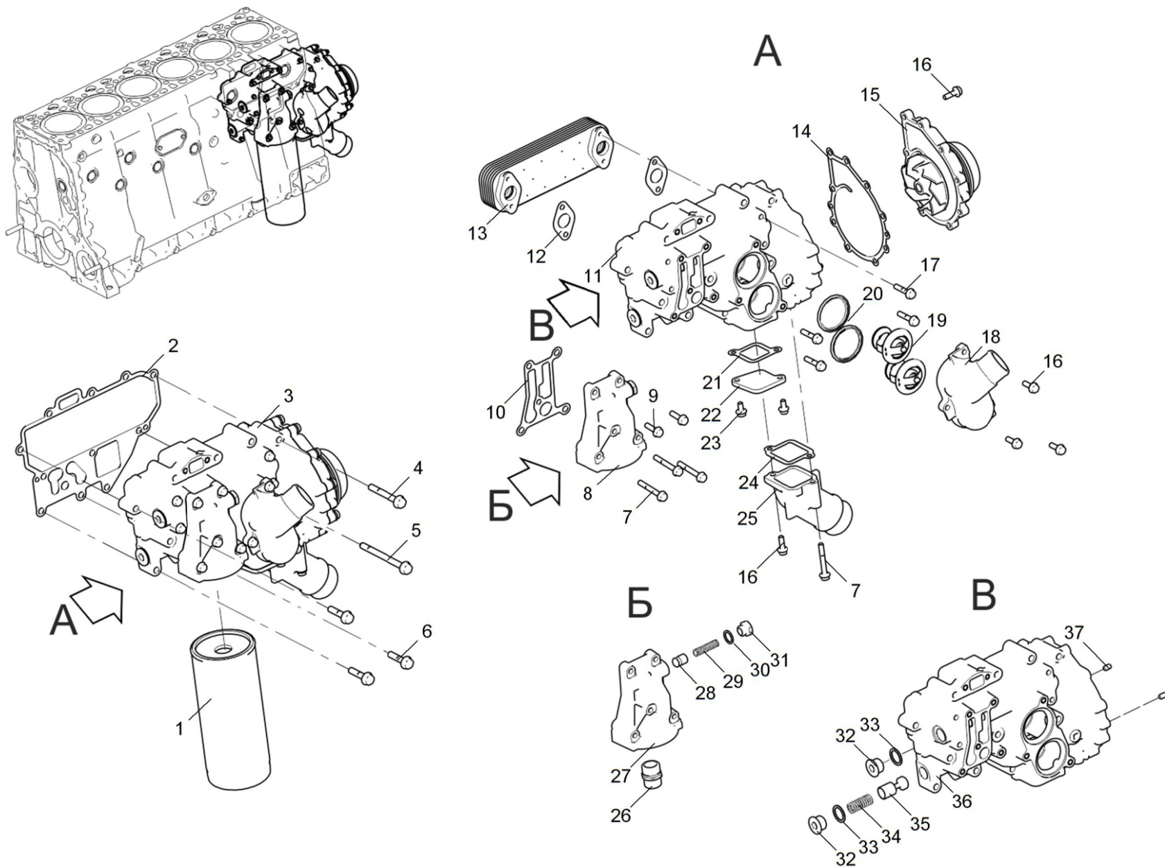
Рисунок 1 Модуль сервисный
