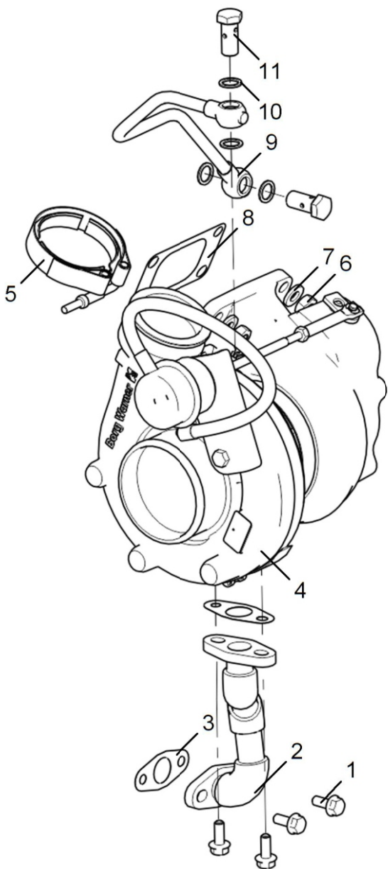
Рисунок 1 ТКР
