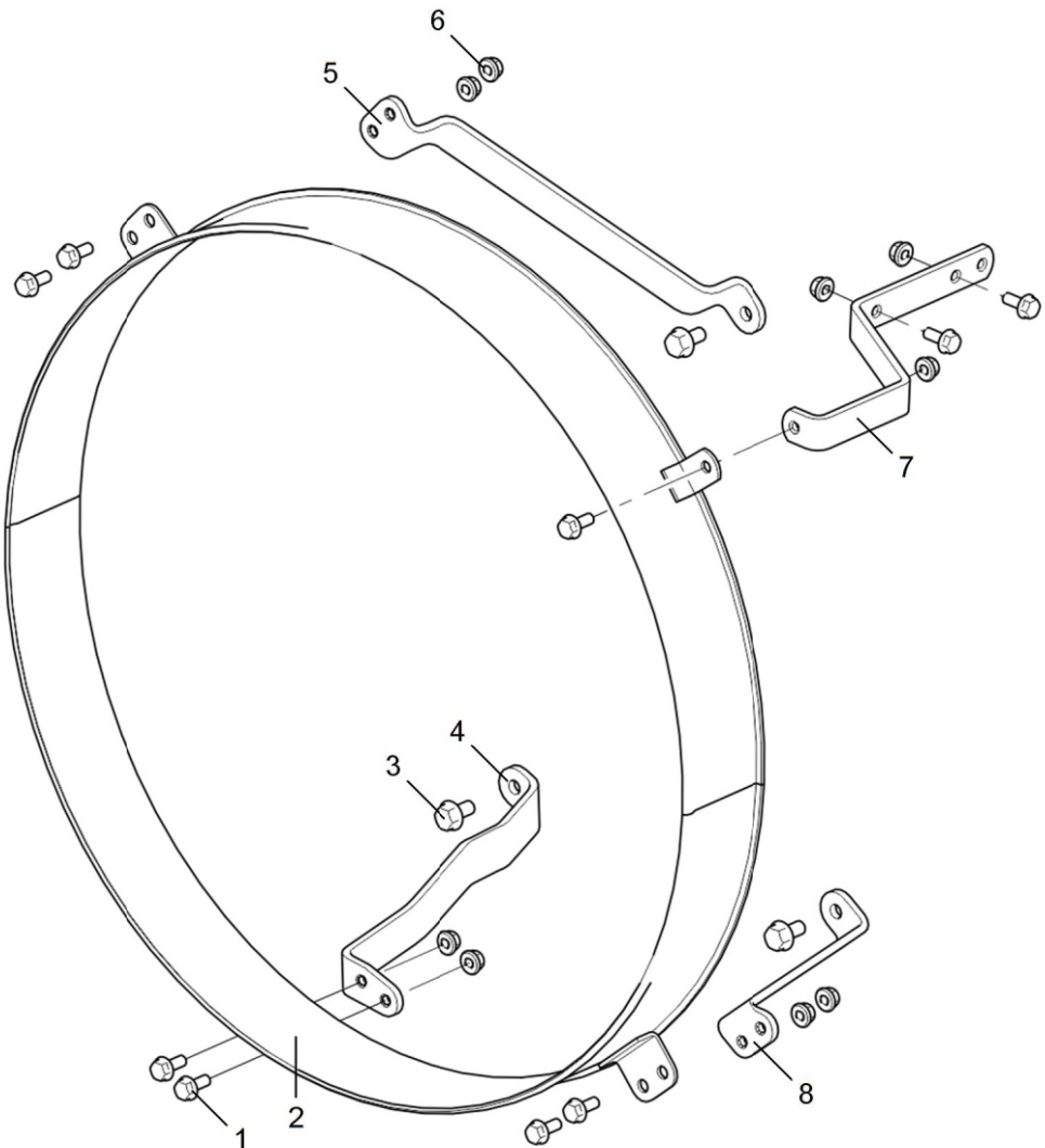
Рисунок 1 Кожух вентилятора
