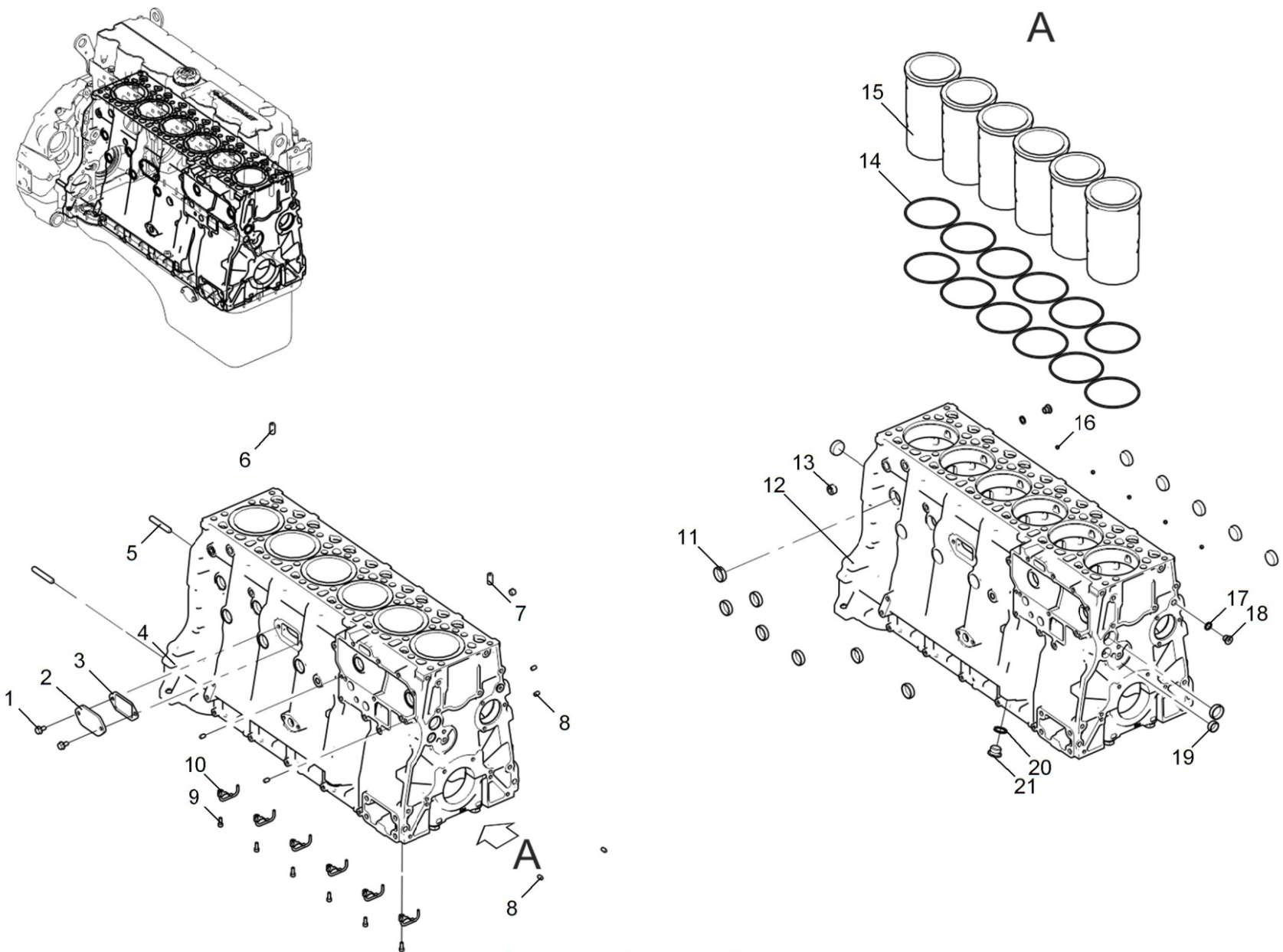
Рисунок 1 Блок цилиндров
