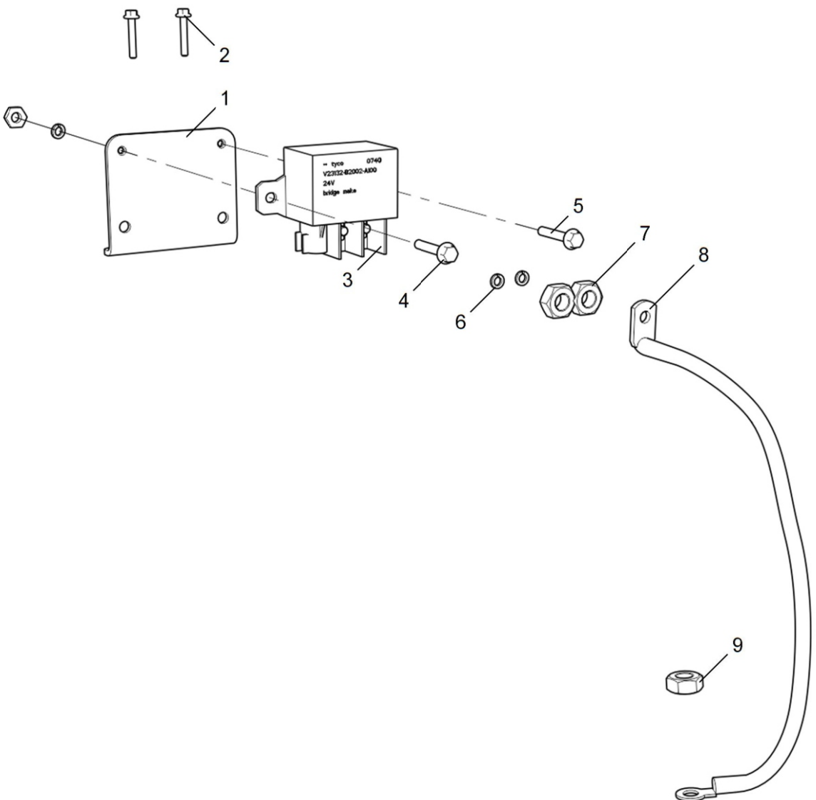
Рисунок 1 Реле подогреватель
