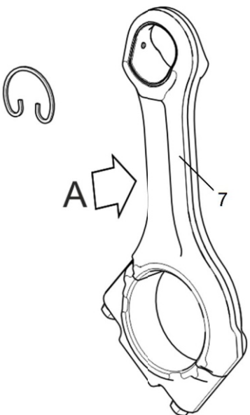
Рисунок 1 Группа шатунно-поршневая
