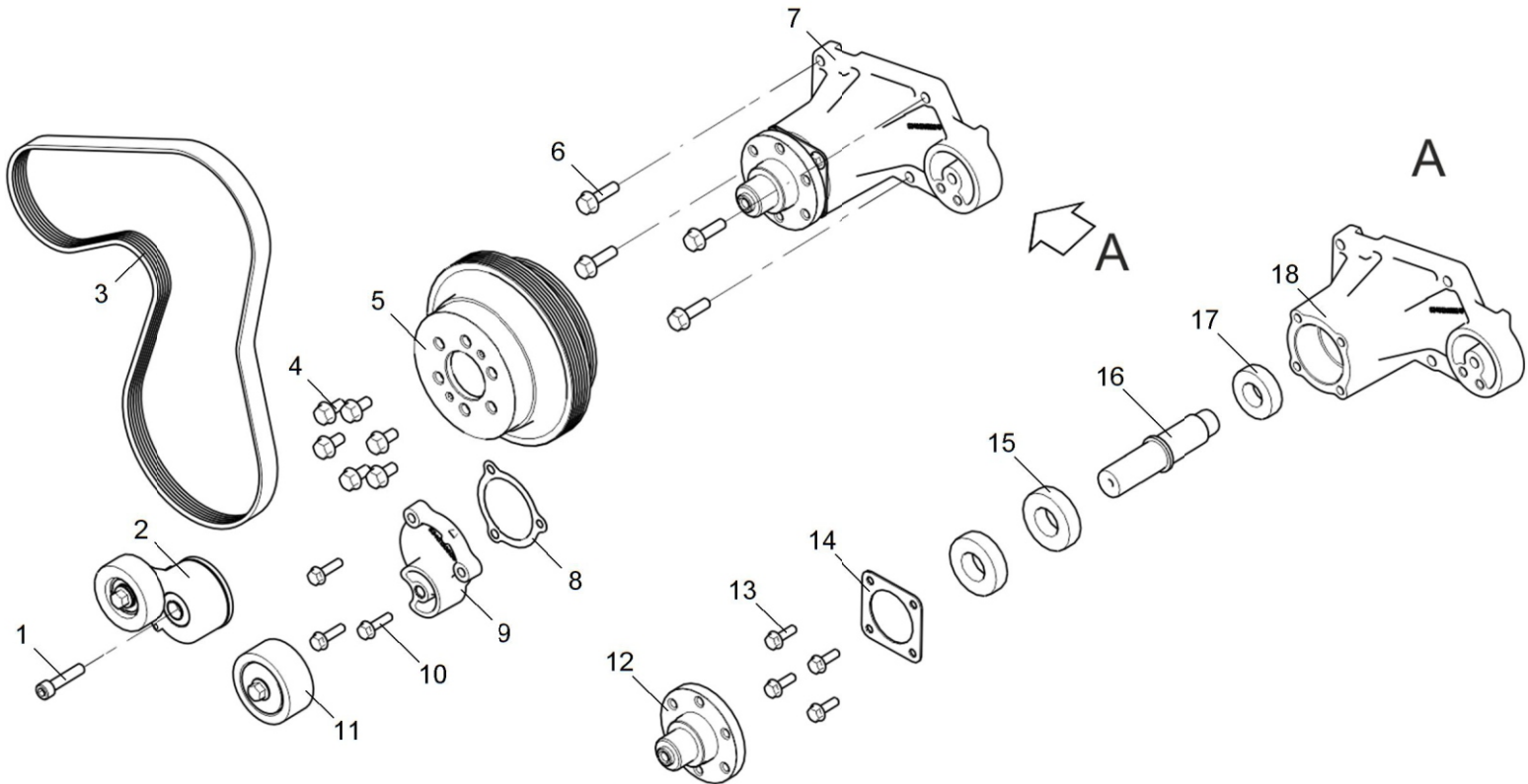
Рисунок 1 Привод вентилятора
