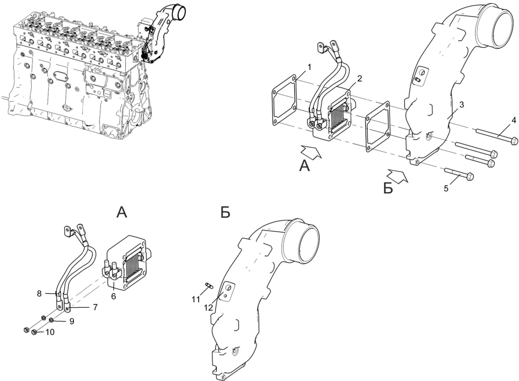
Рисунок 1 Тракт впускной
