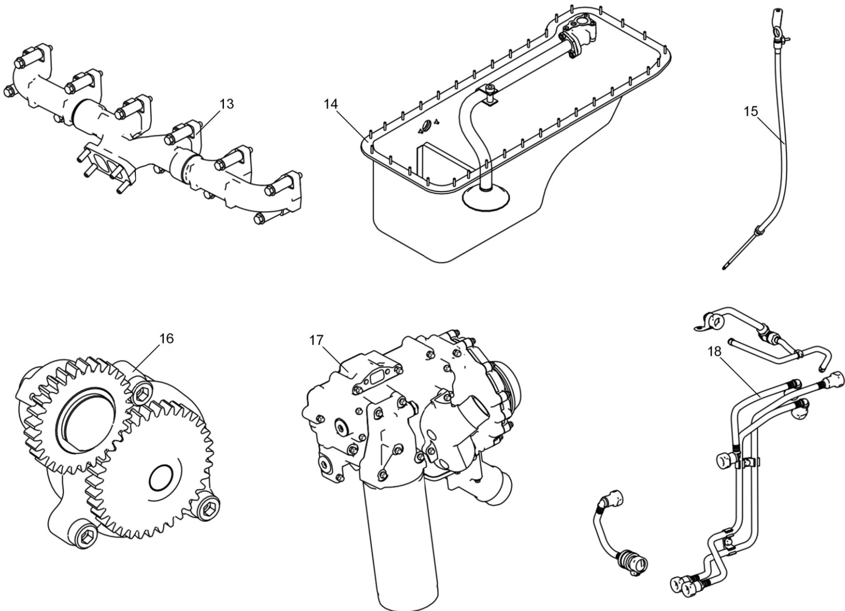
Рисунок 1 Схема деления двигателей ЯМЗ-53602-10, ЯМЗ-53622-10, ЯМЗ-53642-10 на сборочные единицы (Лист 3 из 7)
