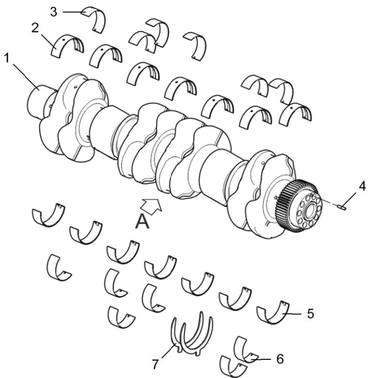
Рисунок 1 Вал коленчатый
