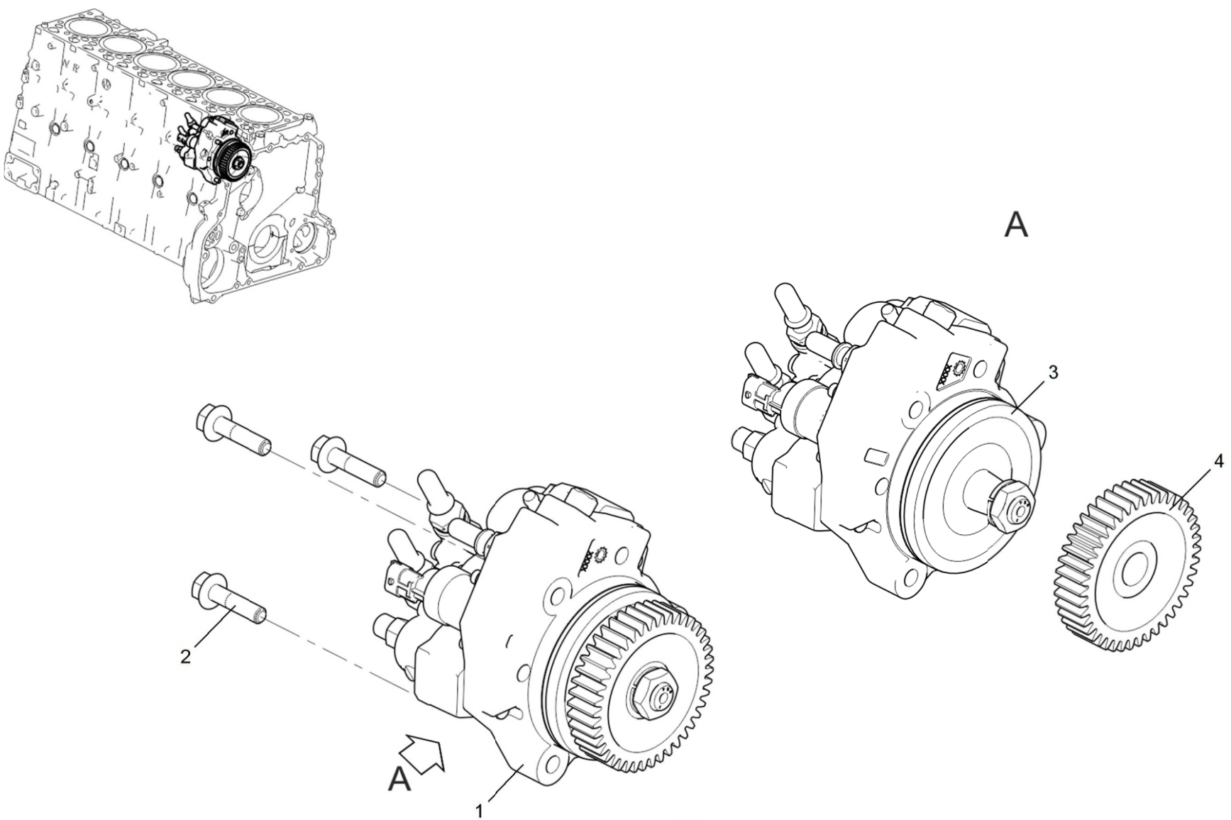
Рисунок 1 ТНВД
