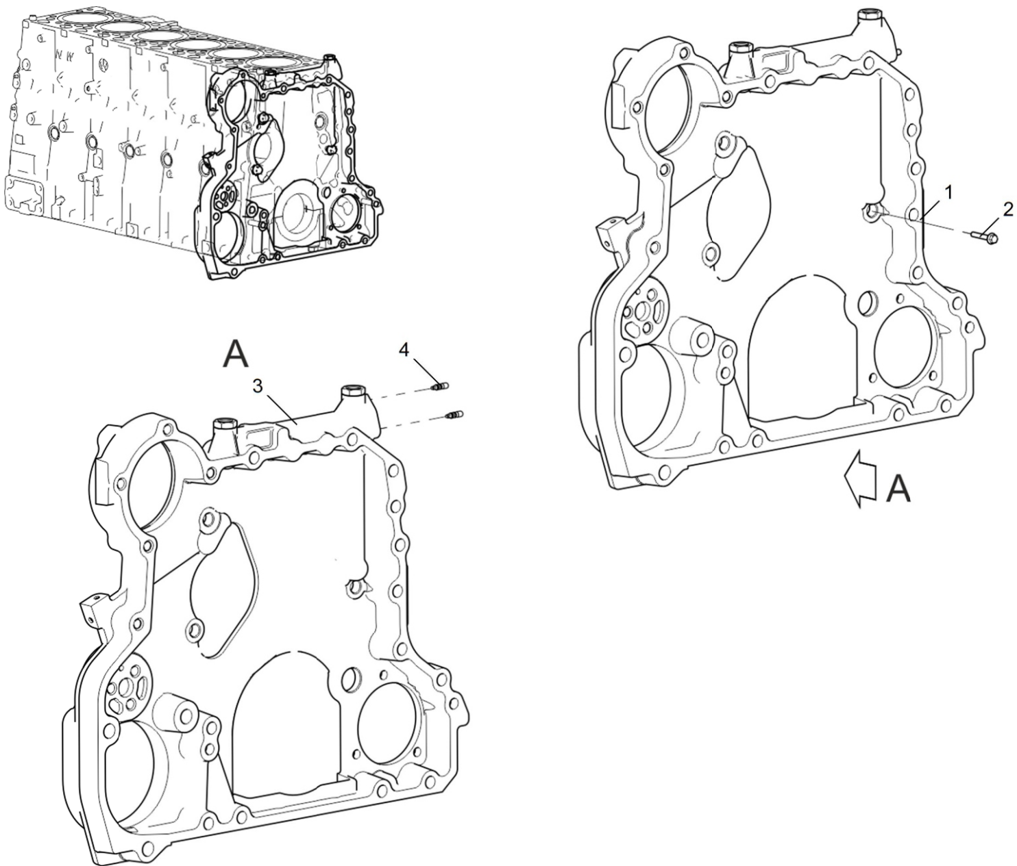
Рисунок 1 Корпус шестерен
