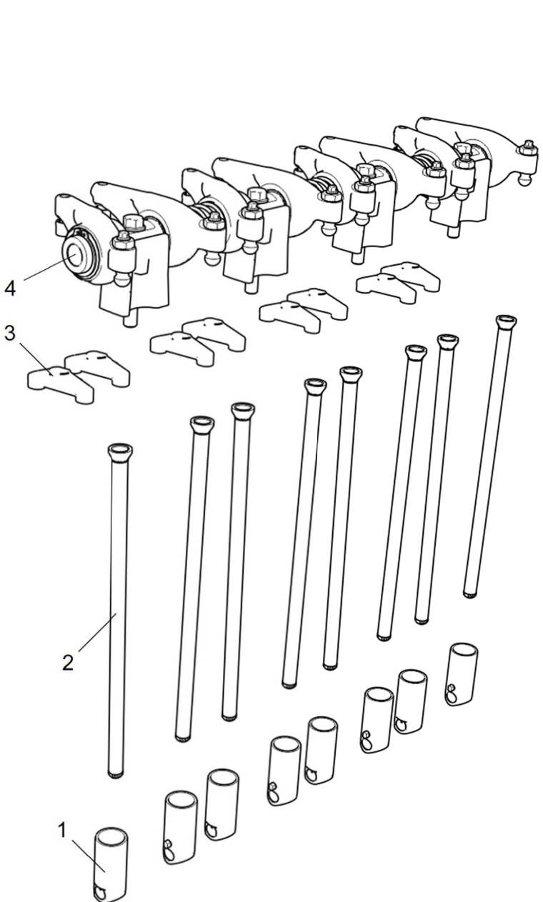
Рисунок 1 Привод клапанов
