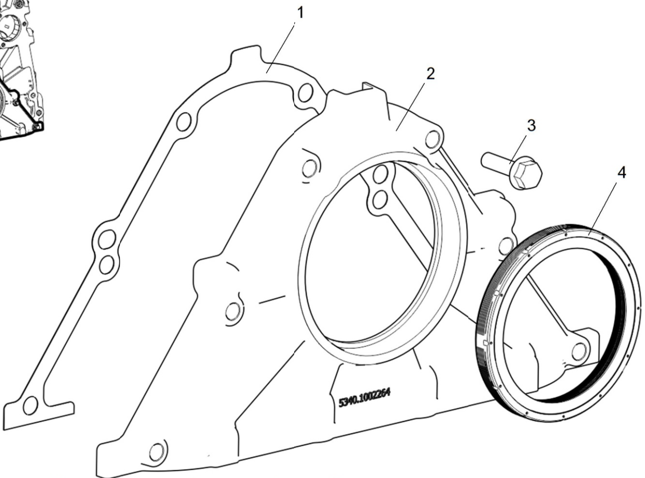
Рисунок 1 Крышка блока цилиндров передняя
