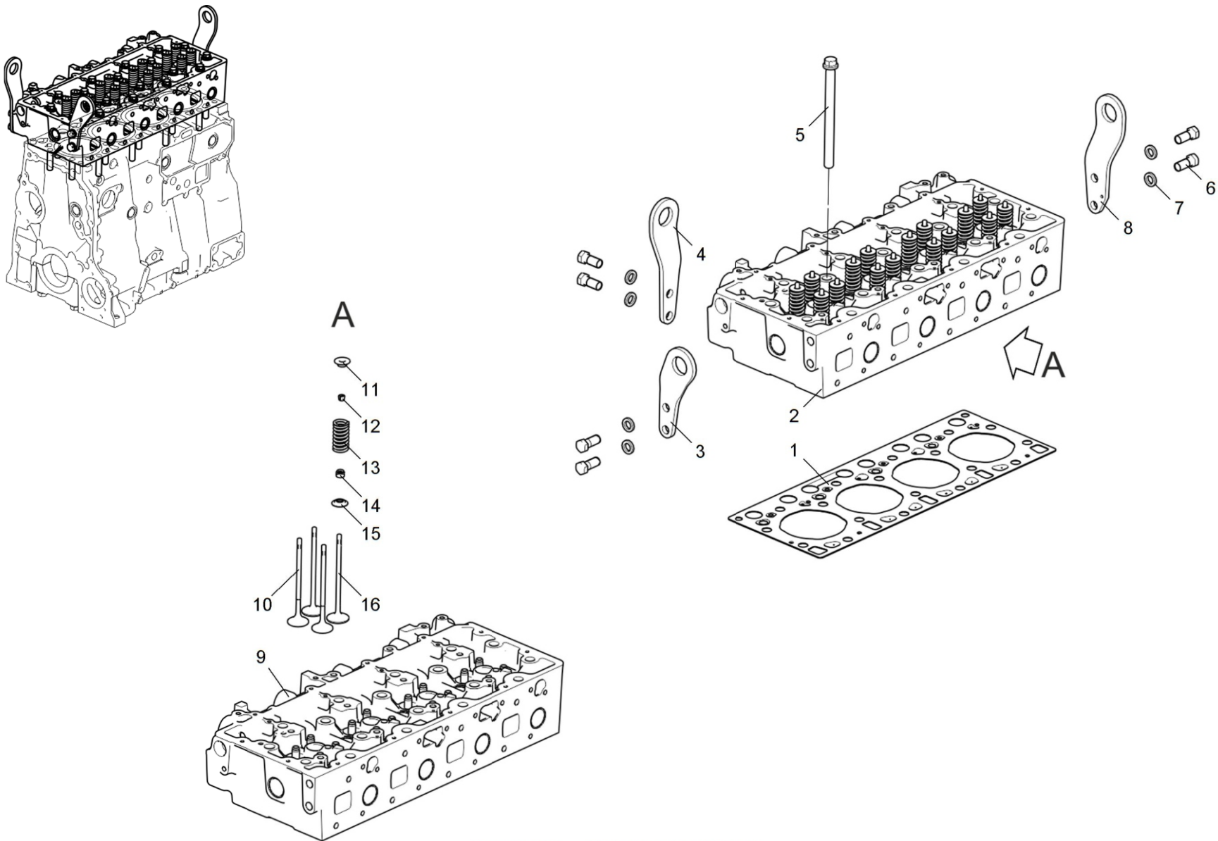
Рисунок 1 Головка цилиндров
