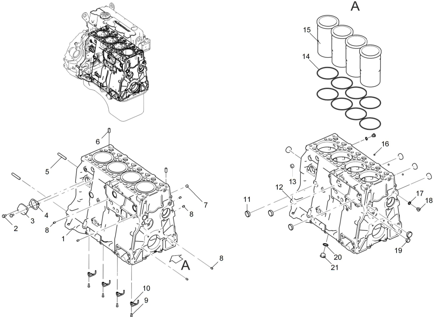
Рисунок 1 Блок циліндрів
