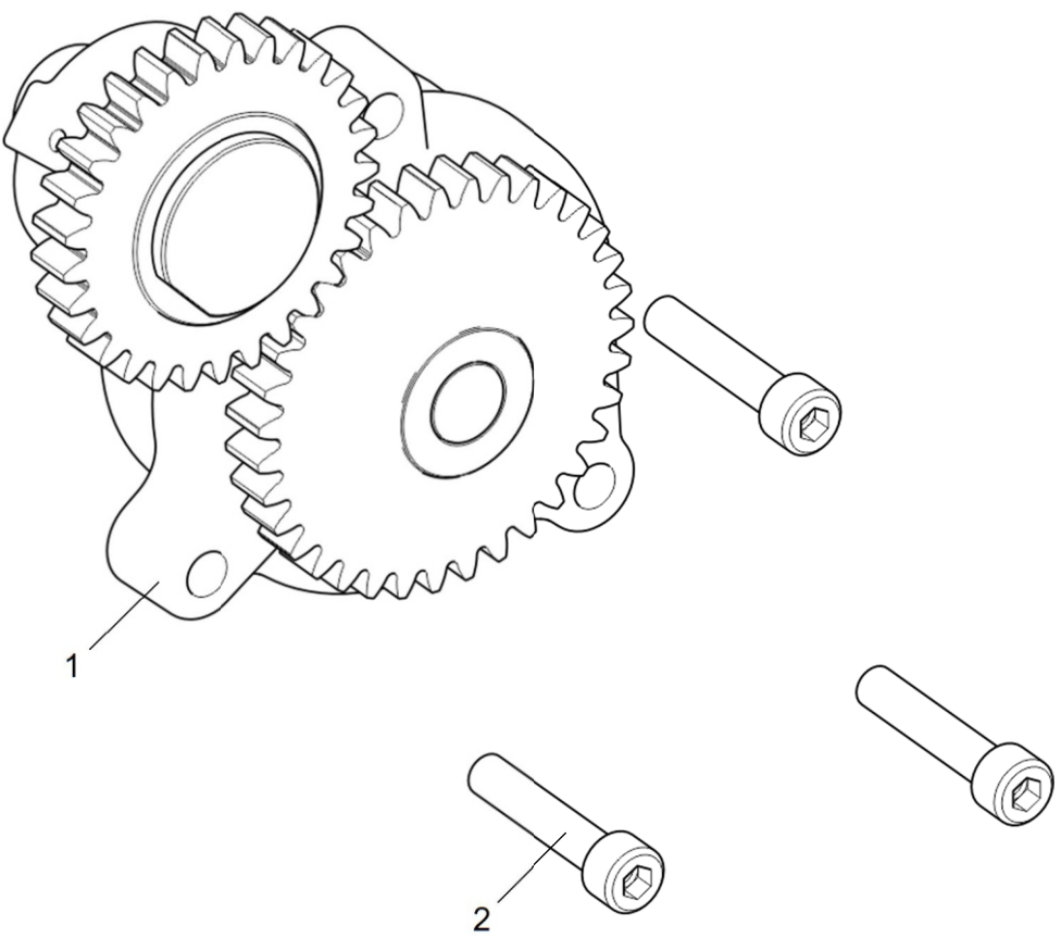
Рисунок 1 Насос масляный
