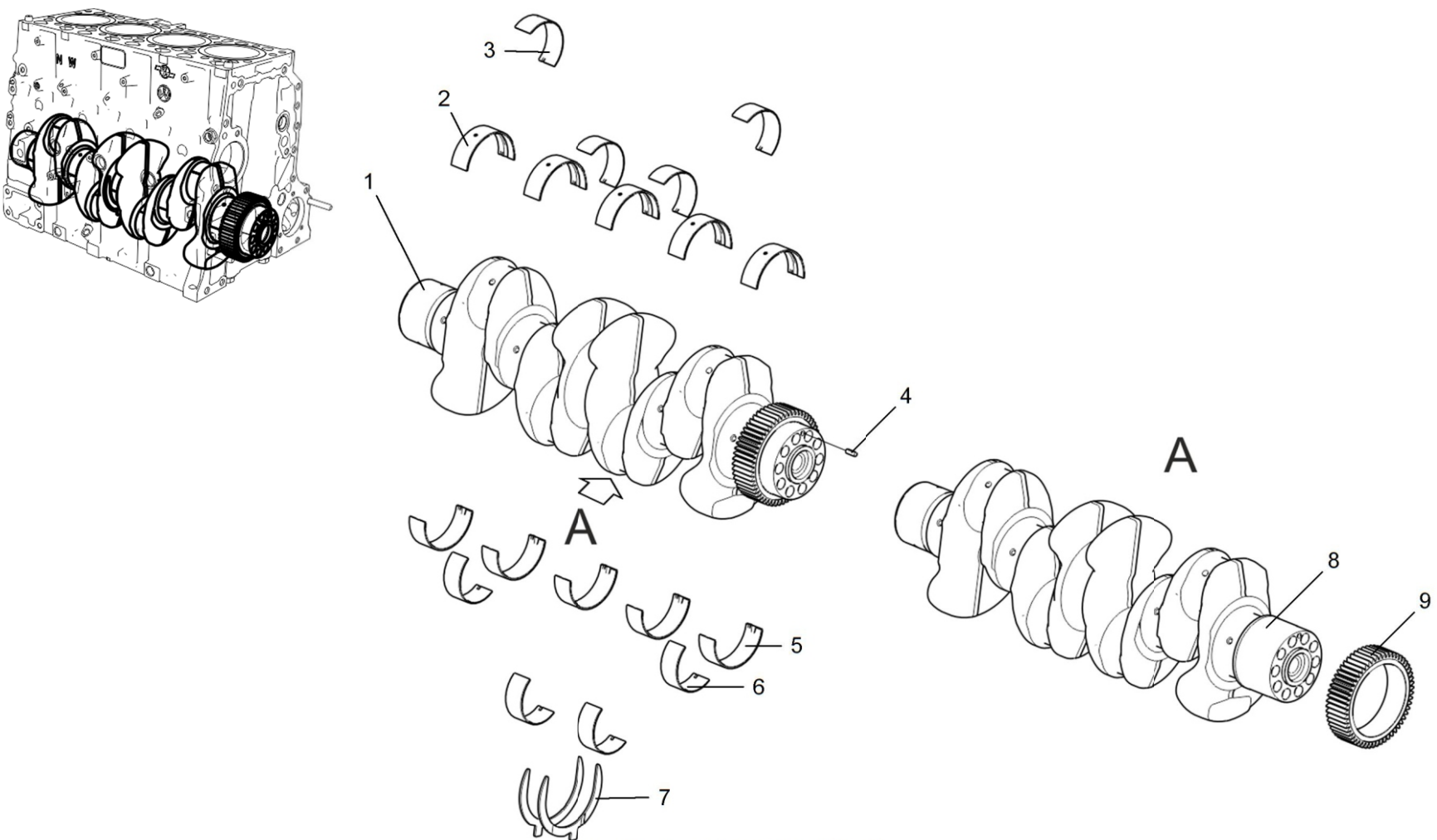
Рисунок 1 Вал коленчатый
