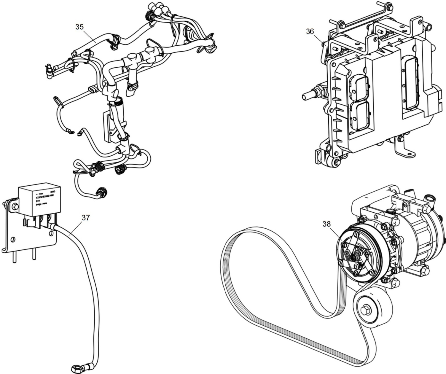
Рисунок 1 Схема деления двигателя ЯМЗ-5341-10 на сборочные единицы (Лист 7 из 7)
