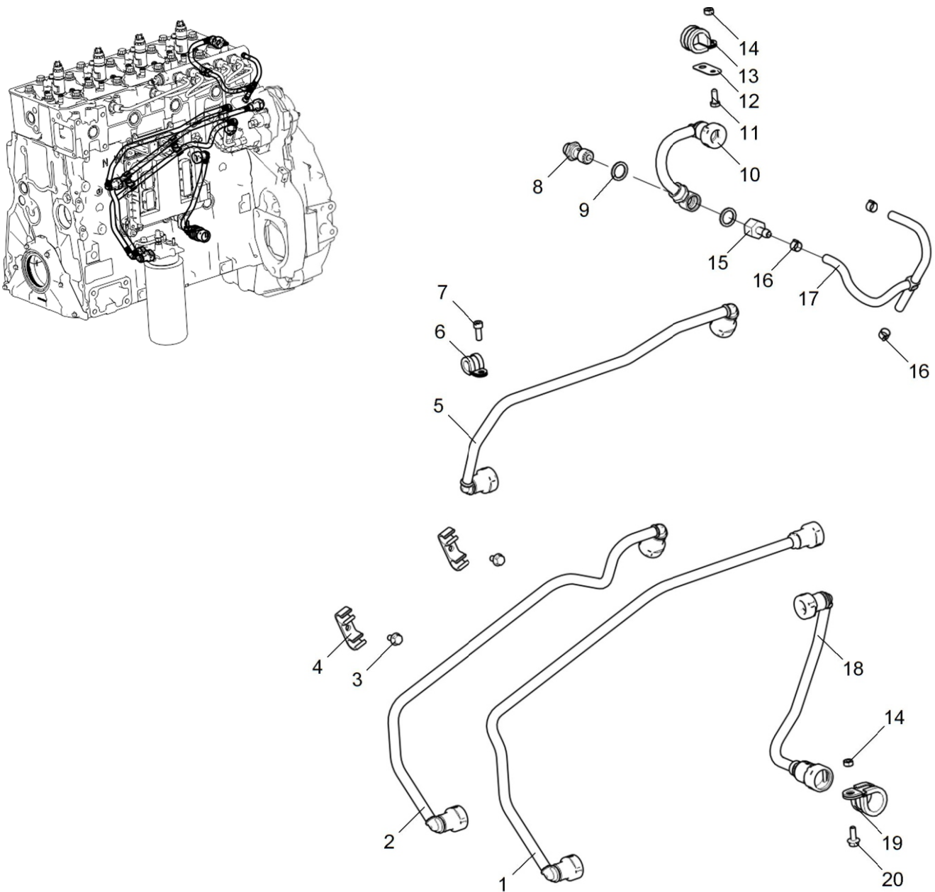
Рисунок 1 Трубопроводы топливные
