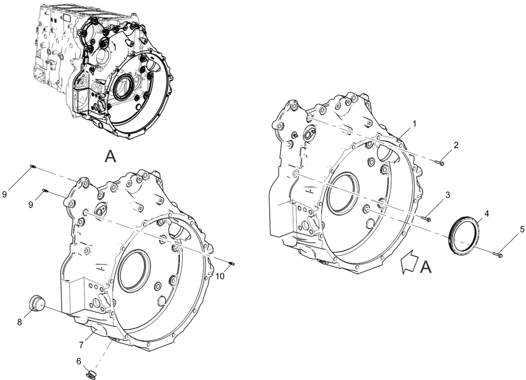
Рисунок 1 Картер маховика
