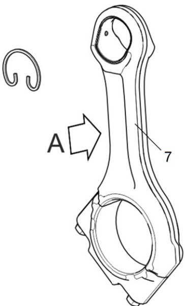
Рисунок 1 Группа шатунно-поршневая
