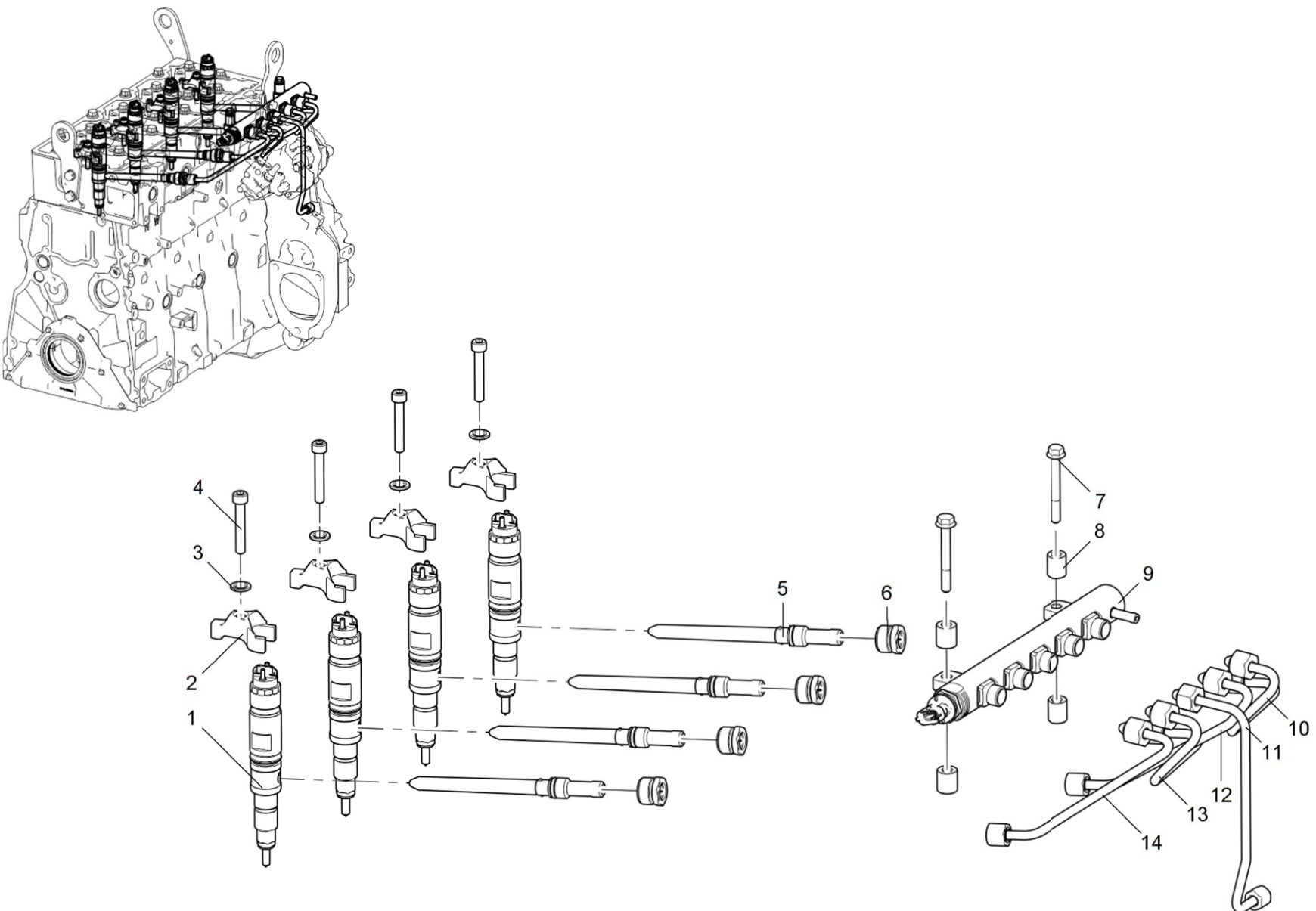
Рисунок 1 Форсунки
