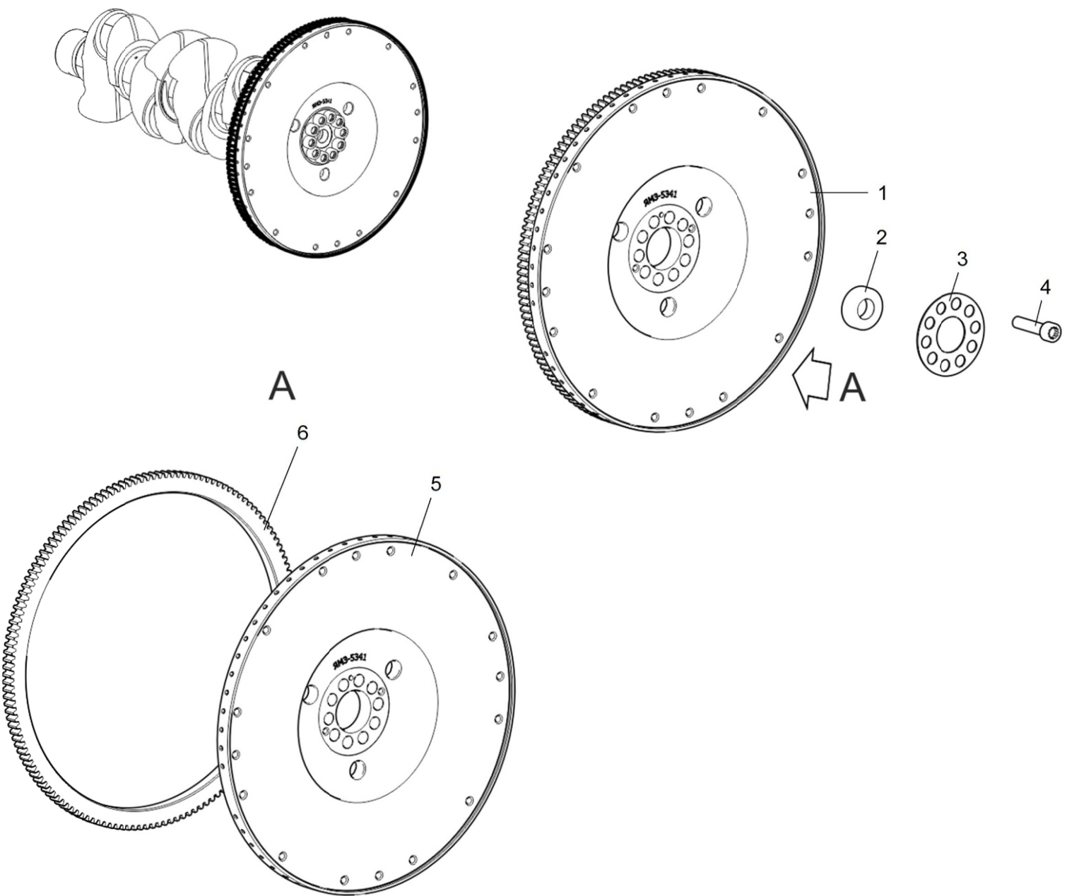
Рисунок 1 Маховик
