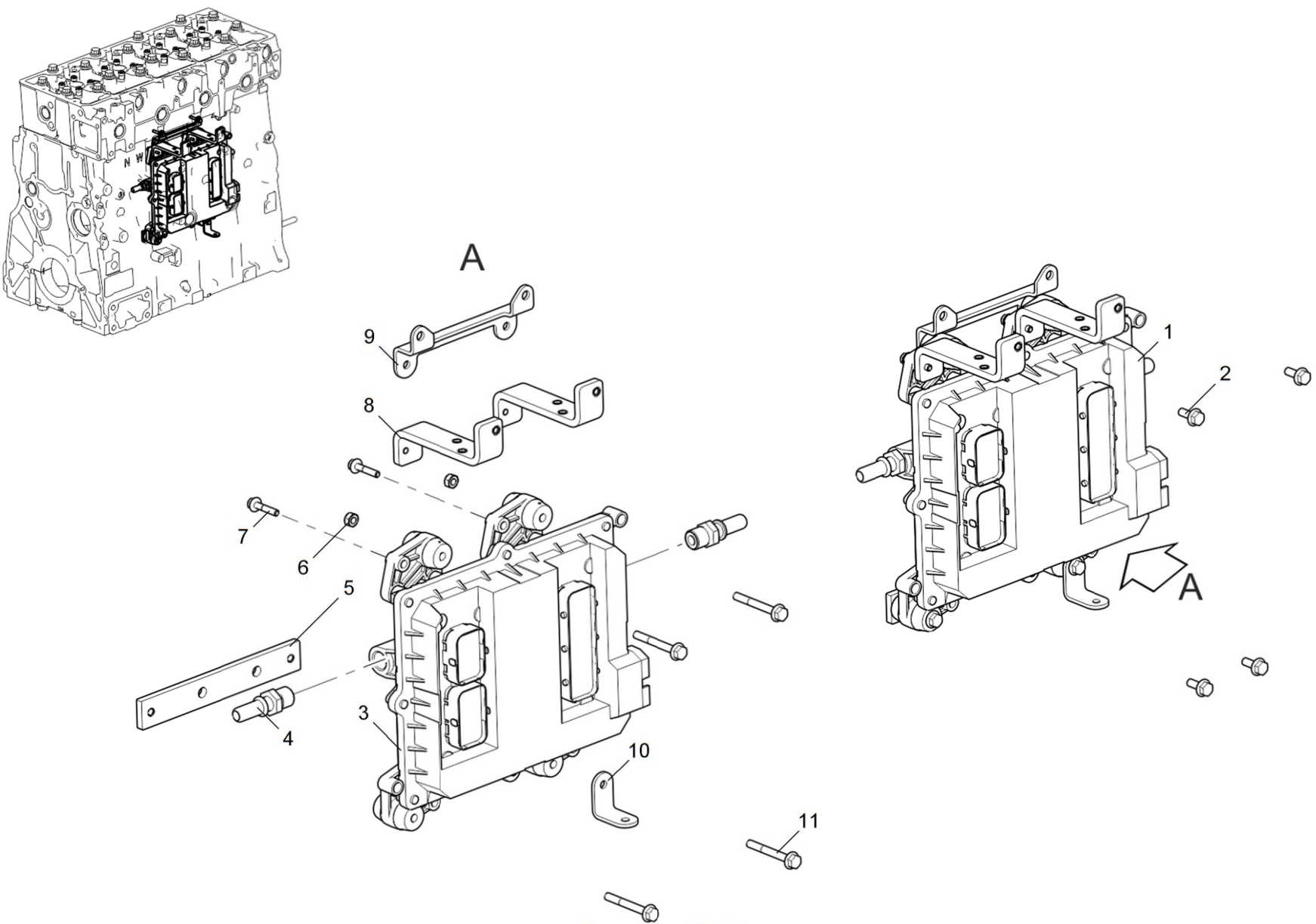
Рисунок 1 ЭБУ
