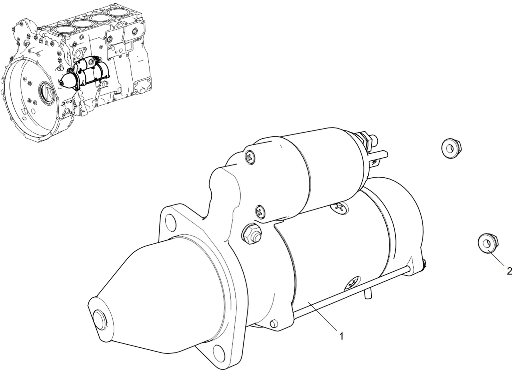
Рисунок 1 Стартер
