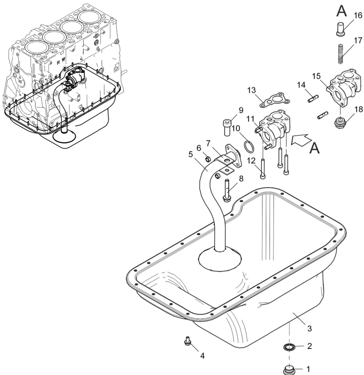
Рисунок 1 Картер масляный
