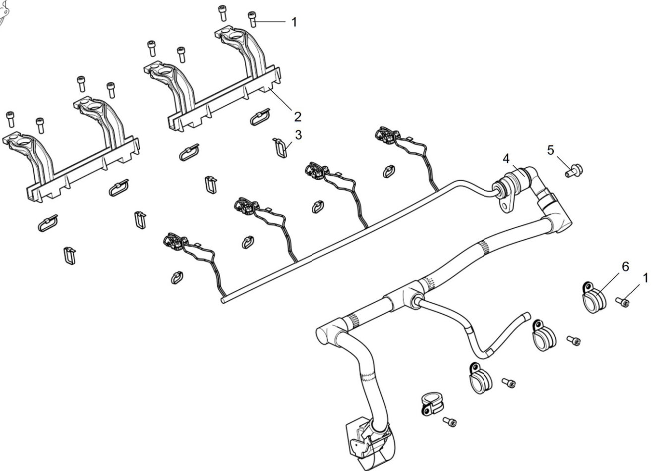
Рисунок 1 Жгут форсунок
