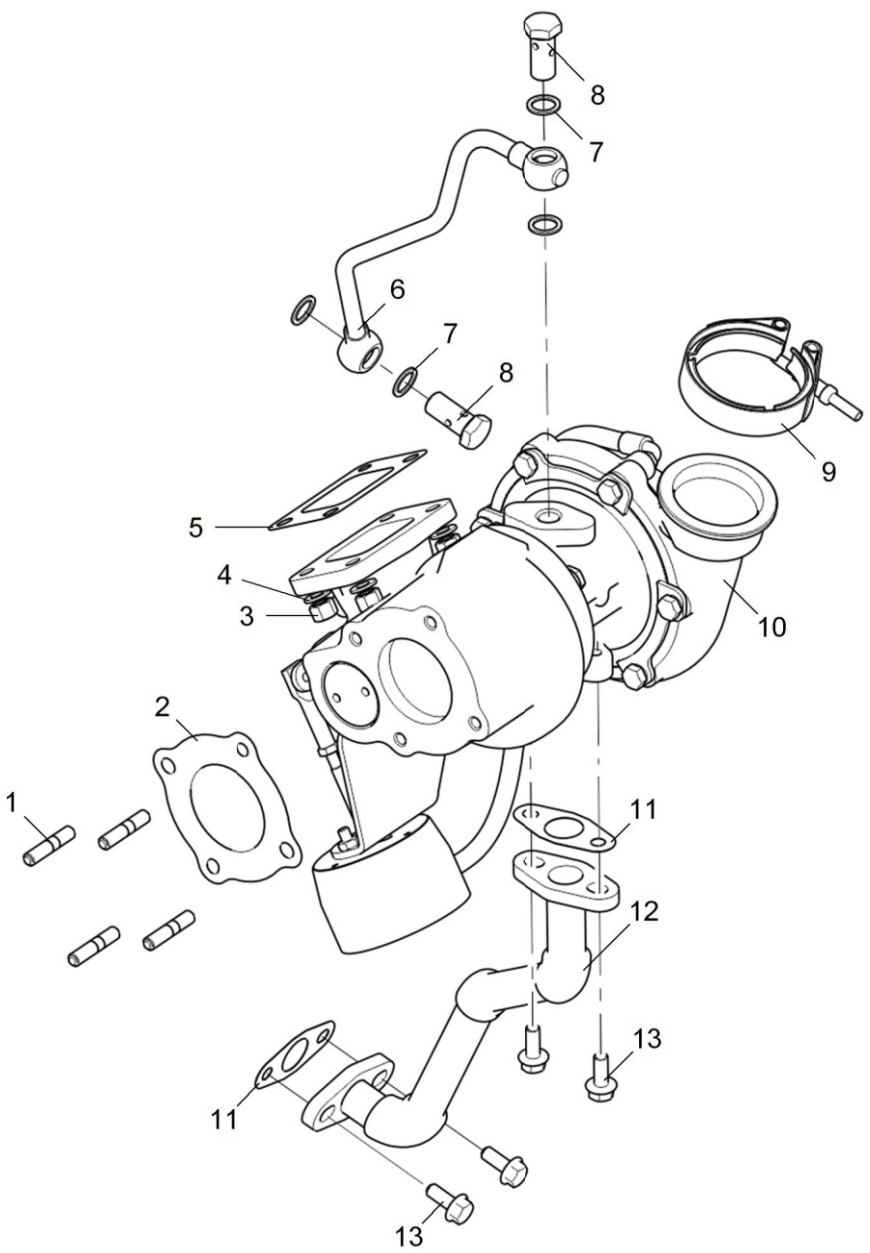
Рисунок 1 ТКР
