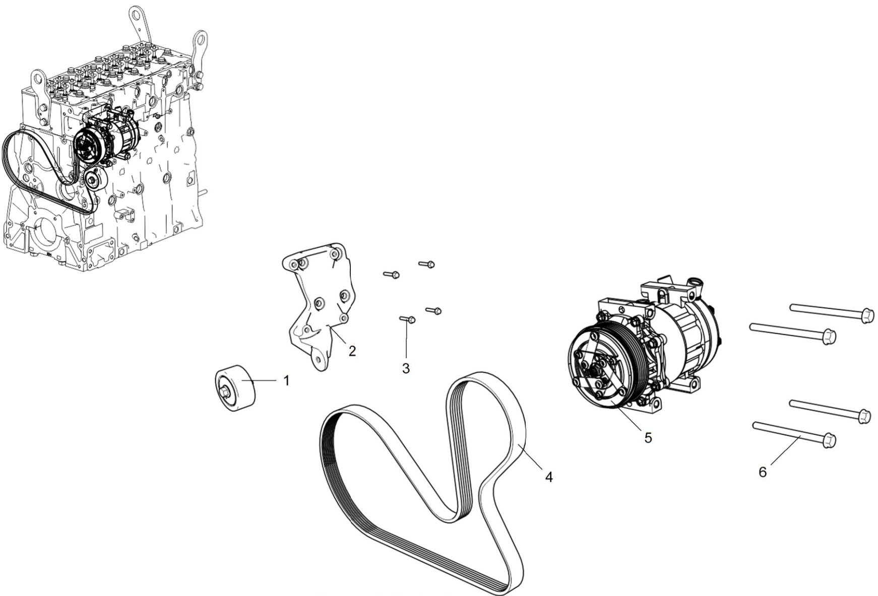
Рисунок 1 Компрессор кондиционера
