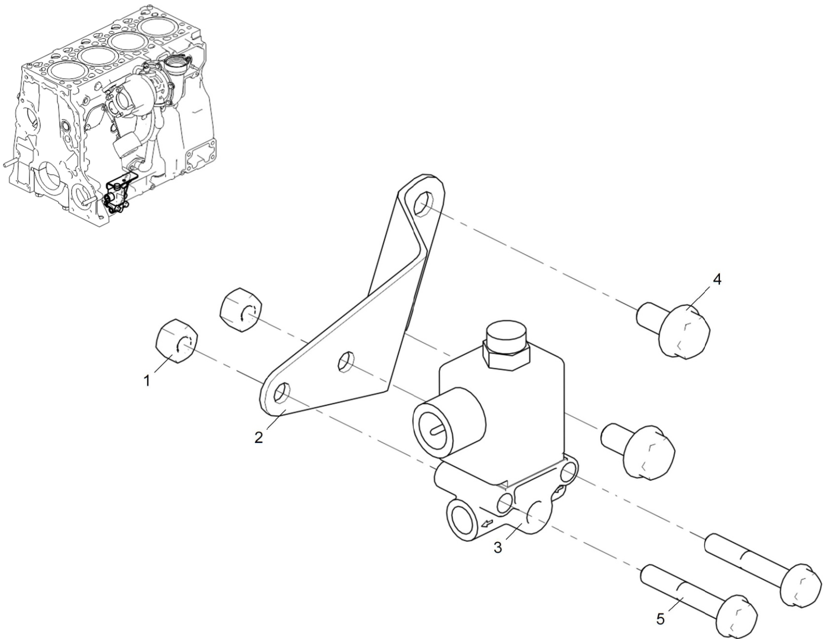
Рисунок 1 Тормоз моторный
