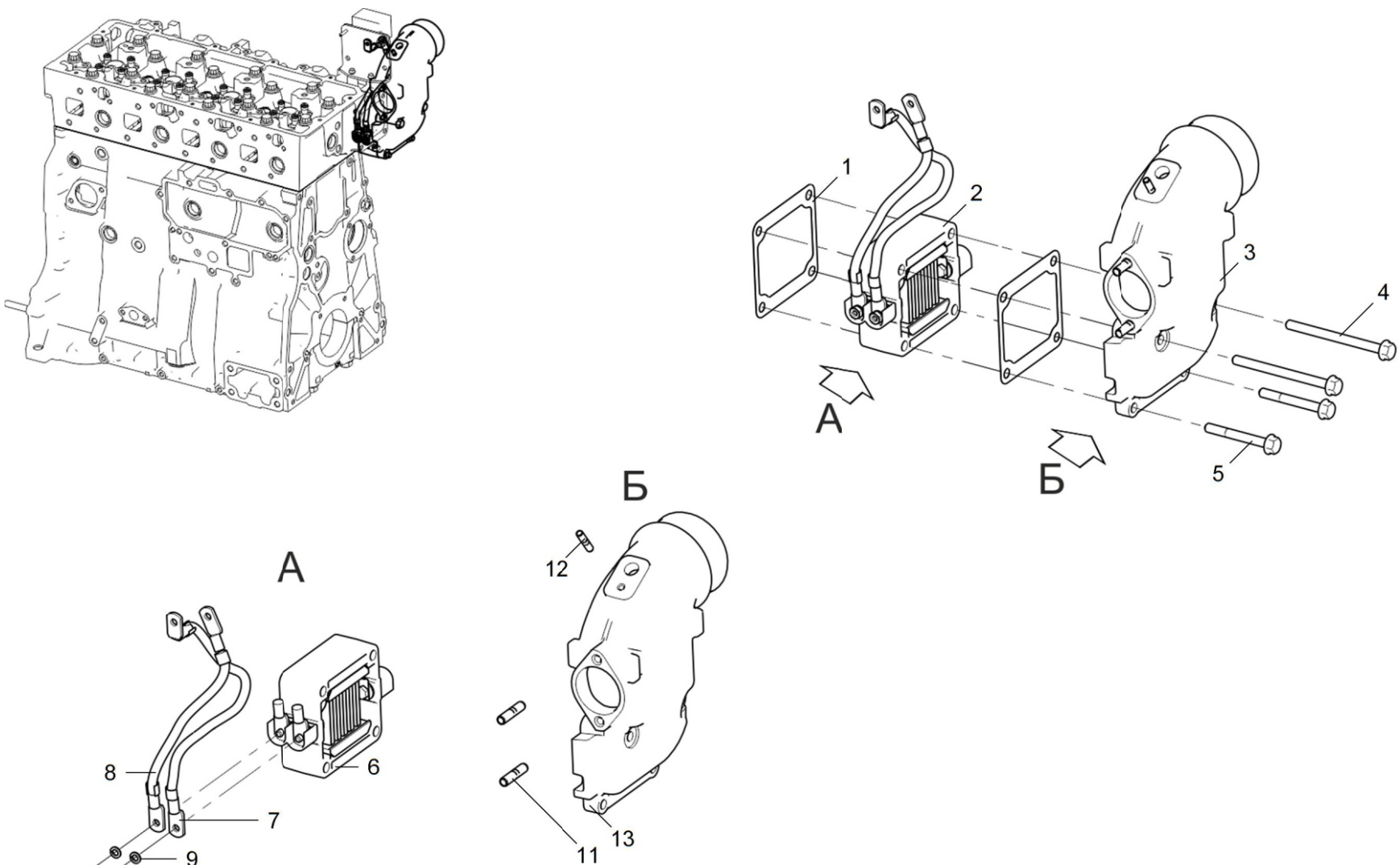
Рисунок 1 Тракт впускной
